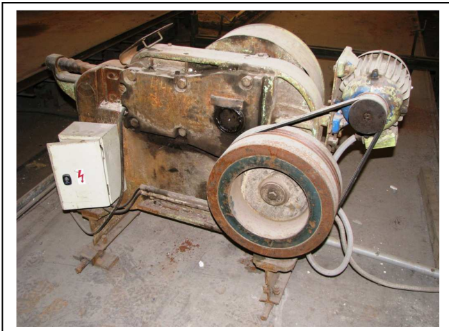
Stříhačka betonářské oceli
